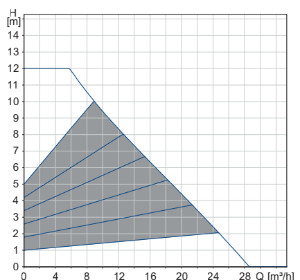
MAGNA3 40-120 F
