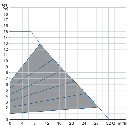
MAGNA3 40-150 F
