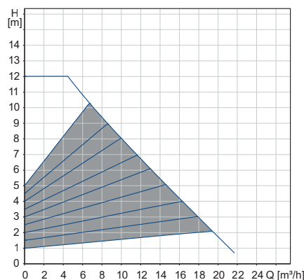
MAGNA3 32-120 F
