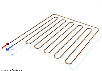
Riviputkitus
