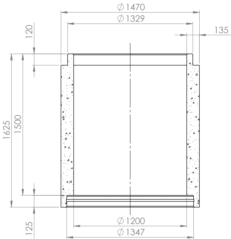
KESKILINJAN LEIKKAUS
