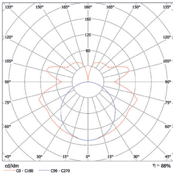
2 X 36 W MAXILUX ST RUNKOVALAISIN
