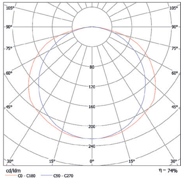
2 X 36 W MAXILUX ST MAALATTU HEIJASTIN
