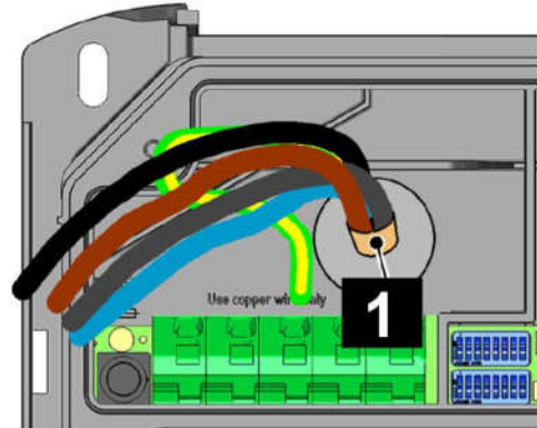
Kaksoiskalvoputki (johdon uppoasennus)
