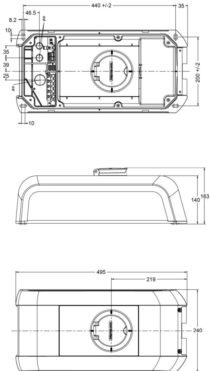
Kuva 12-20: Mitat millimetreinä
