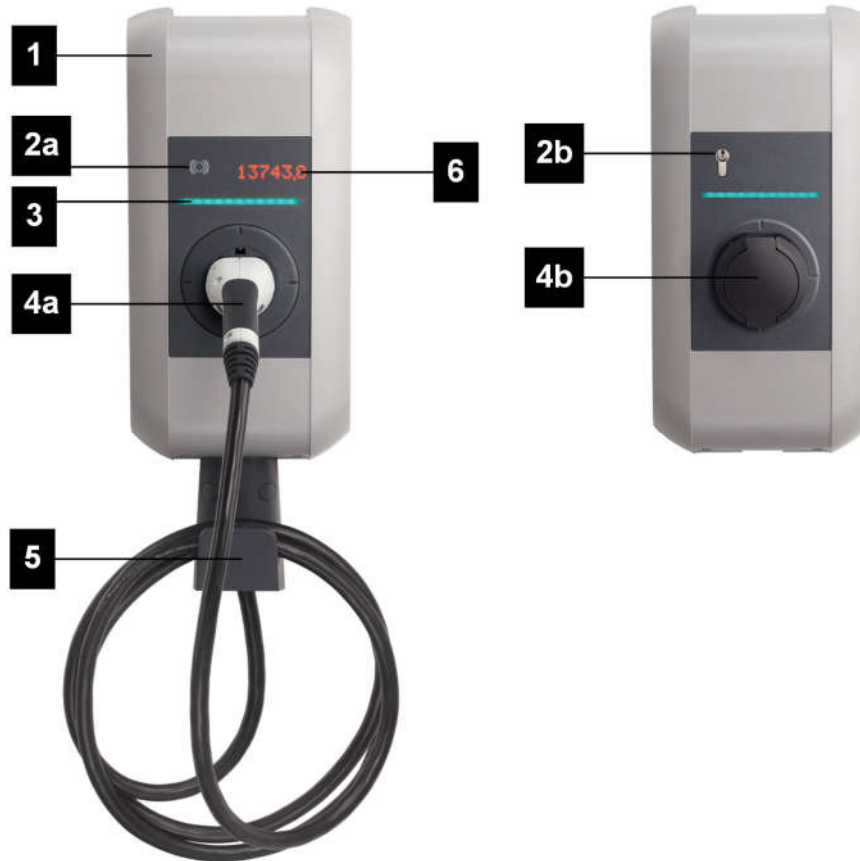
Kuva 4-4: Latausaseman yleiskuva
