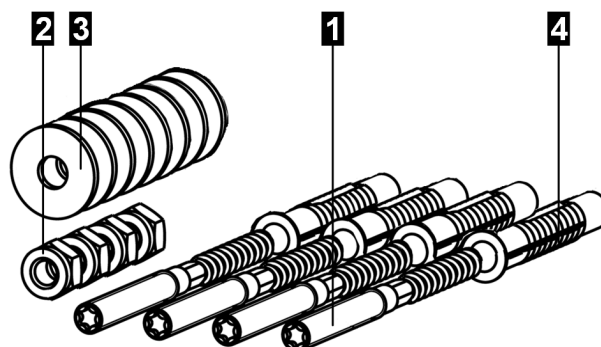
Kuva 3-3: Asennussarja seinäasennukseen
