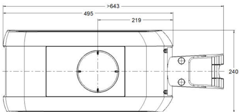
Kuva 12-21: Mitat millimetreinä
