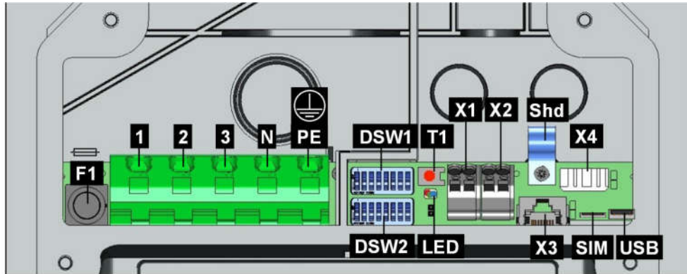
Kuva 7-15: Liitäntöjen yleiskatsaus
