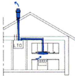
Tulo/poisto-järjestelmässä
