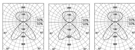
1x32/35 W, kapea runko
