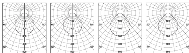
3x13/14 W 4x13/14 W 2x25/28 W 1x25/28 W
