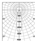
Keskileveä sirontakulma, 3000 lm
