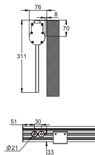
SEINÄASENNUS TW802XX+TW77503
