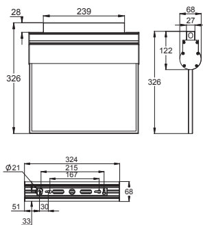
KATTOASENNUS TW802XX+TW77501
