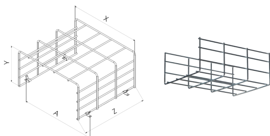
PALLOSUOJA TW77510B
