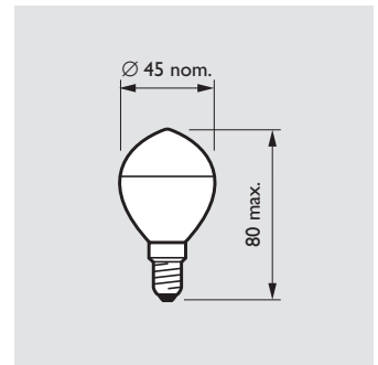
PC45 25W/40W E14
