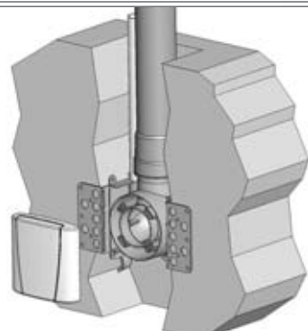
Kiviseinäasennus
