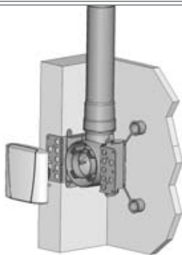
Levyseinäasennus
