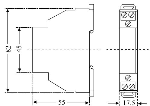
Mittapiirros (mm)
