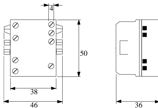
Mittapiirros (mm)
