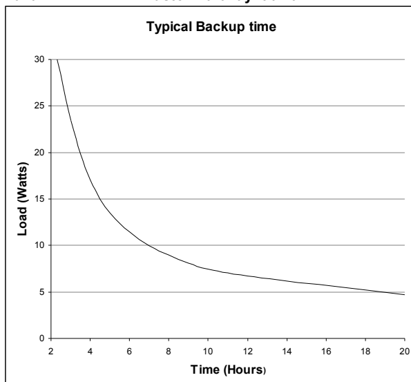
Kuva 1: 12V/7Ah Akuston varakäyntiaika
