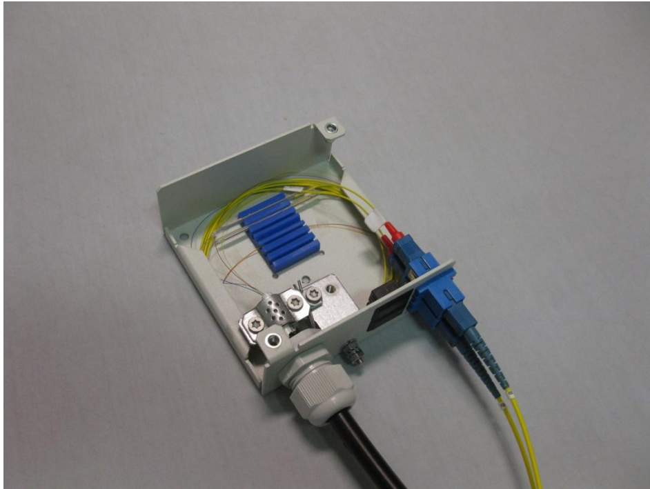
Päätekotelo NC-125 asennettuna
