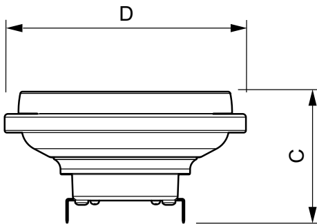
AR111 12V 15W-75W 890lm 40D 4000K G53 D
