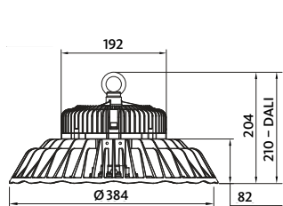
AURA CERTOS 200 W & 240 W
