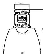
Valaisin symmetrisellä heijastimella.
