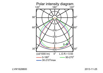
IFPC1_TBS460 SQR 3xTL5-14W HFP C8-VH.EPS
