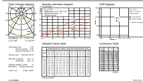
IFGU1_TBS460 SQR 2xTL5-14W HFP C8.EPS
