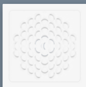
ARIES-2 (DYCH)
