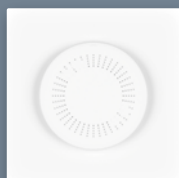
ATLAS-4 (RPPH)
