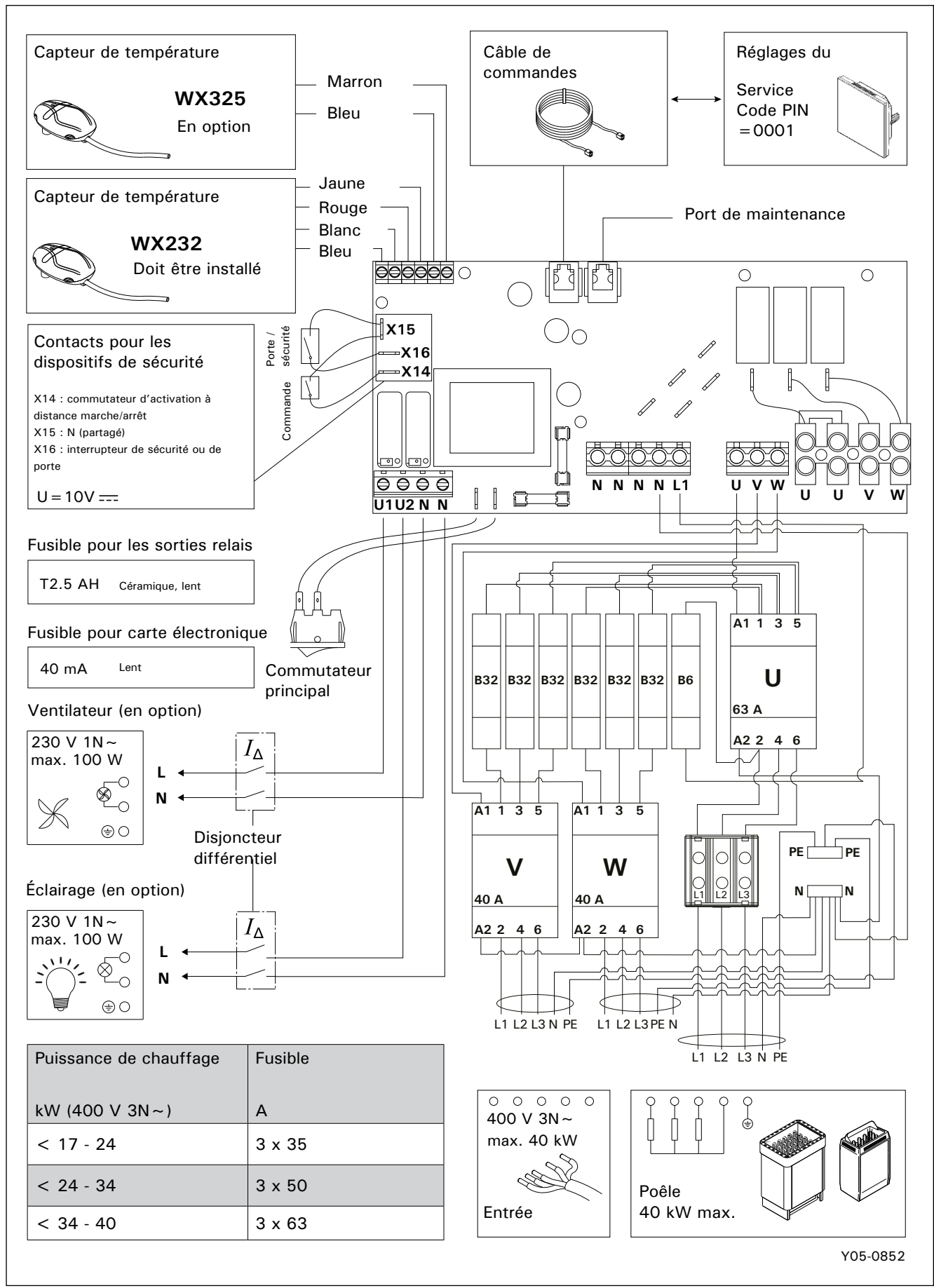
Figure 8. Raccordements électriques
