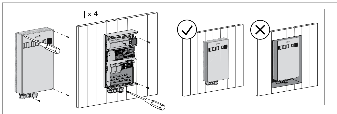
Figure 7. Ouverture du couvercle du bloc d'alimentation et montage du bloc au mur
