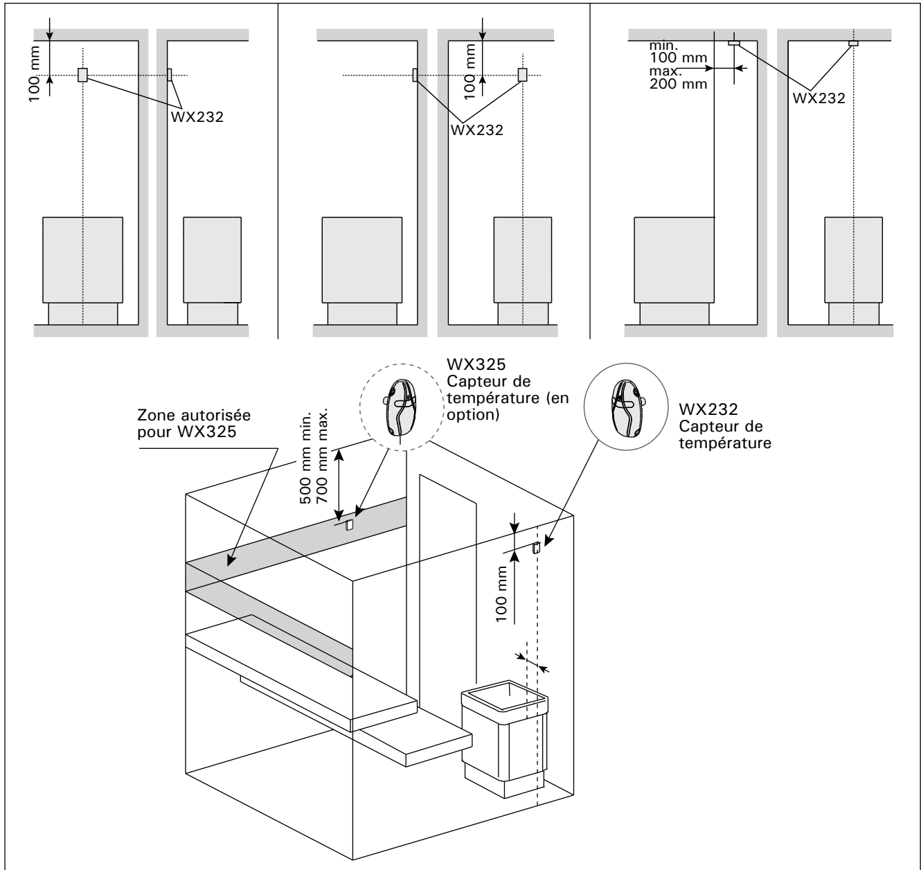
Figure 10. Emplacement des capteurs de température pour les poêles au sol
