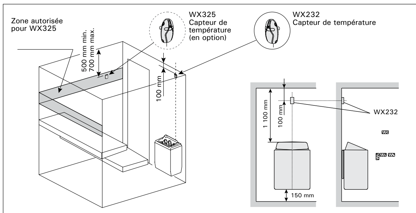
Figure 9. Emplacement des capteurs de température pour les poêles muraux
