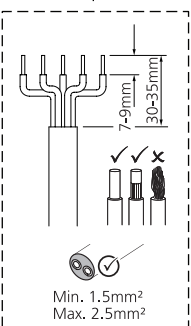
4b(iv) 220-240V~ + DALI
