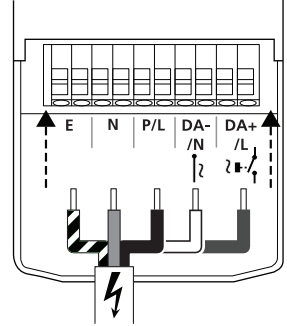
4b(iii) 220-240V~ + DALI
