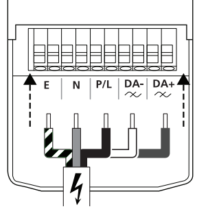
4b(iii) 220-240V~ + DALI
