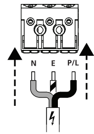
3b 220-240V~ + DALI
