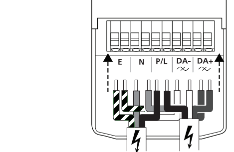
4b(iv) 220-240V~ + DALI
