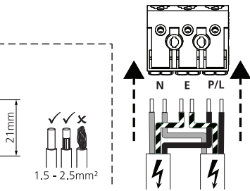
4b(i) 220-240V~ + Switch-Dim
