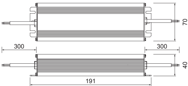
4016048 Tasajännitelähde 24V 100W IP67 DIM
