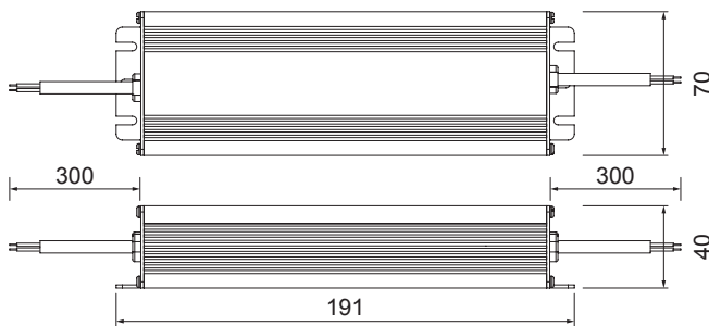
4016049 Tasajännitelähde 24V 150W IP67 DIM
