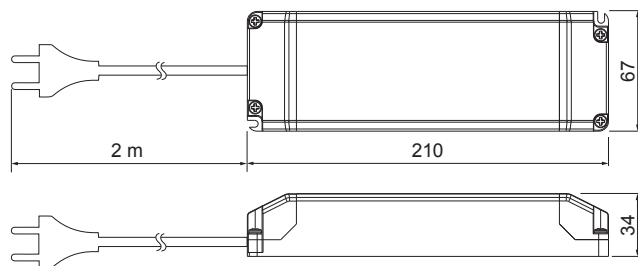
4016045 Tasajännitelähde 24V 150W IP20 DIM
