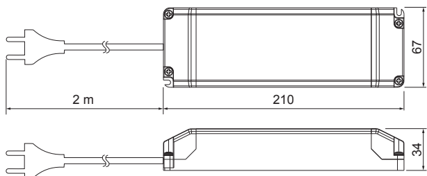
4016044 Tasajännitelähde 24V 100W IP20 DIM
