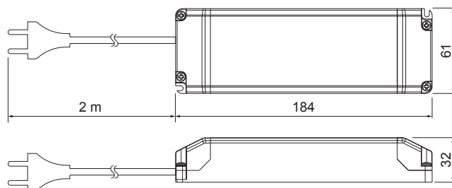
4016043 Tasajännitelähde 24V 50W IP20 DIM
