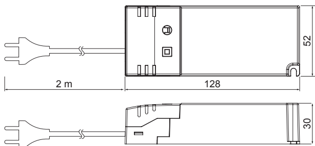
4016042 Tasajännitelähde 24V 25W IP20 DIM
