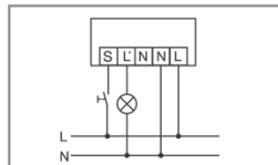
Standardbetrieb mit zusätzlicher Ansteuerung durch einen Taster.
