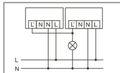
Parallelbetrieb von max. 8 Geräten.
