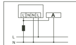
Bei Schaltung von Induktivitäten (z. B. Relais, Schütze, Vorschaltgeräte) kann der Einsatz eines Löschiodes (A) erforderlich sein.
