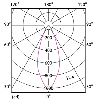
LEDspots MAS 6W PAR20 E27 830 40D
