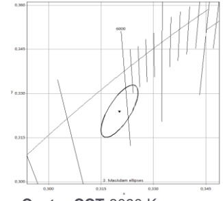
Center CCT 6090 K Cx=0,32 ; Cy=0,32
