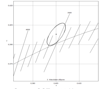
Center CCT 3560 K Cx=0,4 ; Cy=0,4
