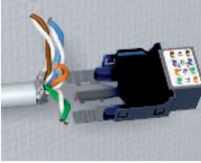
Liittimen kytkentä - kaapelin kuorinta Kaapelin päällyks ja suoja poistetaan 50 mm:n mitalta.
