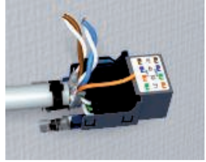
Liittimen kytkentä - parien erottelu Yksittäiset johtimet asennetaan liittintämerkintöjen mukaisesti liittimiin.
