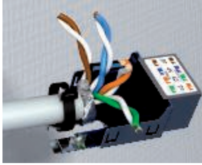
Vedonpoisto Kaapeli työnnetään liittintäkappaleeseen ja vedonpoisto toteutetaan johdinsiteellä. Suojatuissa kaapeleissa on varmistettava, että suojaus on kiinni liittintäpinnassa.
