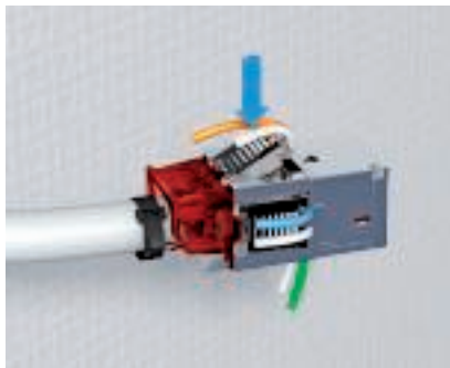
Liittimen kytkentä - päättäminen Liitinliuskat sijoitetaan ja lukitaan liittimen runkoon. Lisäliitimet katkaisevat ylimenevät johdonosat ja ne pitää poistaa.
