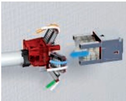
Liittimen kytkentä - osien yhdistäminen Kytkeäosa ja liittinosa painetaan yhteen ja lukitaan. Molemmissa rakennusosissa on asennuksen helpottamiseksi merkintä.
