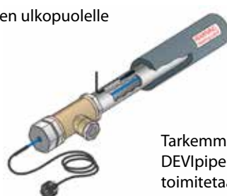
Asennus putken sisäpuolelle
