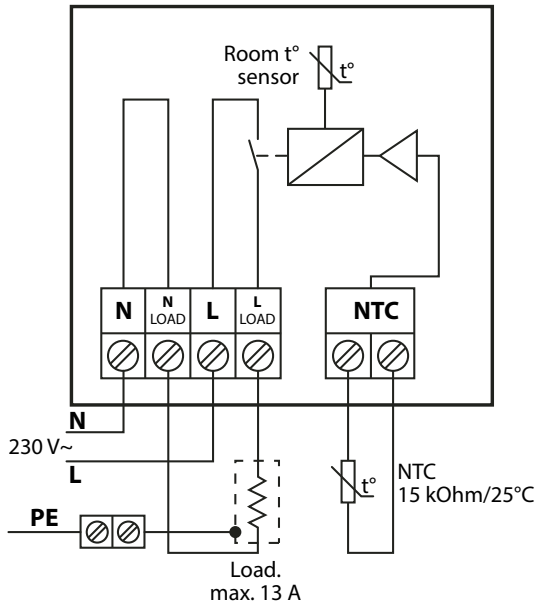
DEVireg™ Smart
