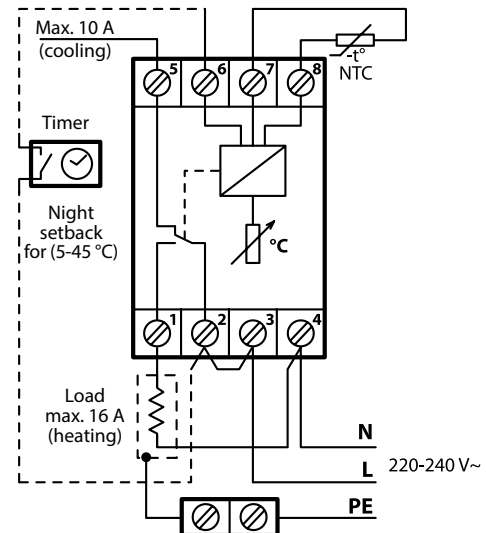
DEVireg™ 330
