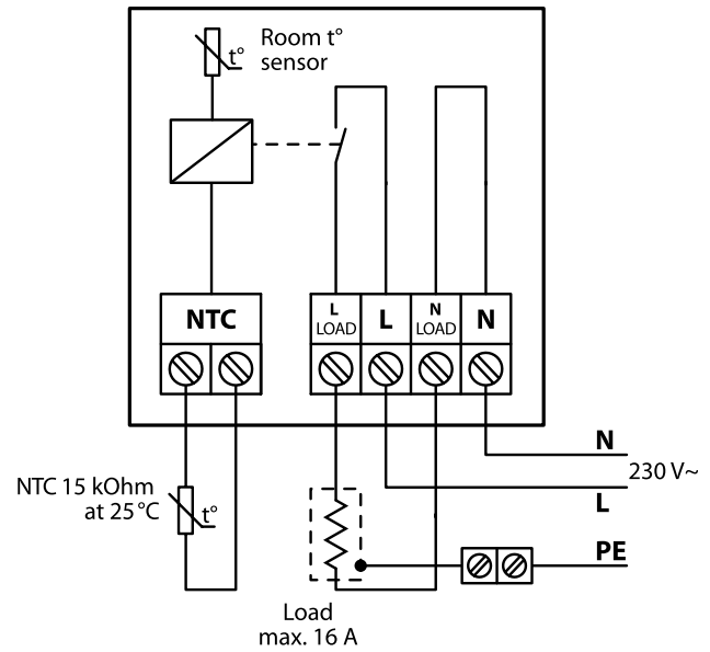
DEVireg™ Touch
