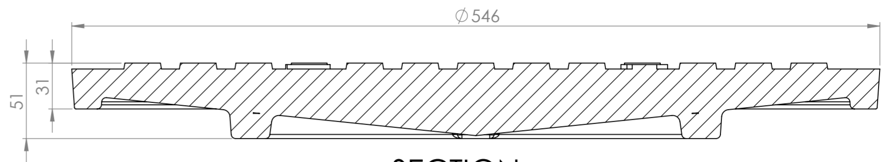
SECTION A-A
