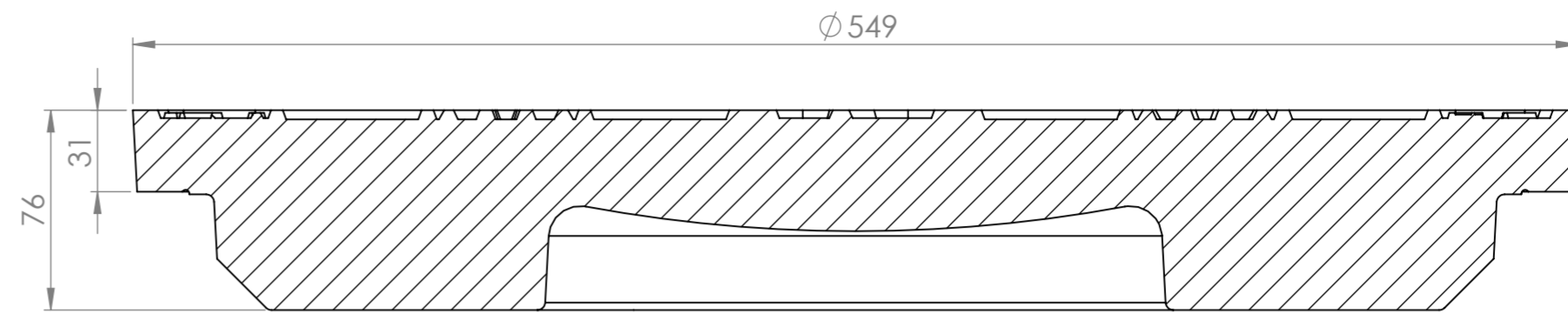
SECTION A-A
