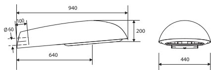
611/612HGV akryylikupu
