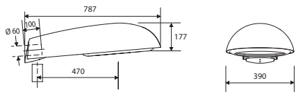
621HGV akryylikupu
