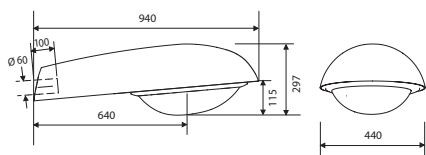
611/612HGV akryylikupu
