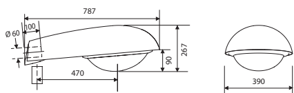
621HGV akryylikupu
