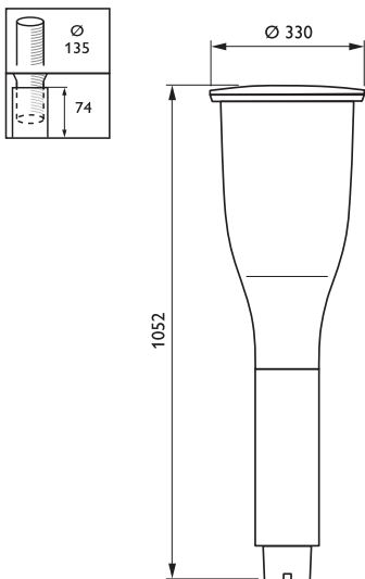
BDS650 GRN40--2S/830 PSR-CLO II MDS 60
