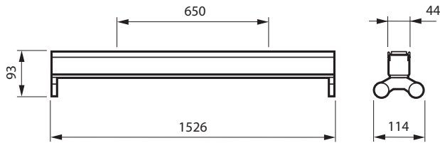
TMX204 2xTL-D58W HFP
