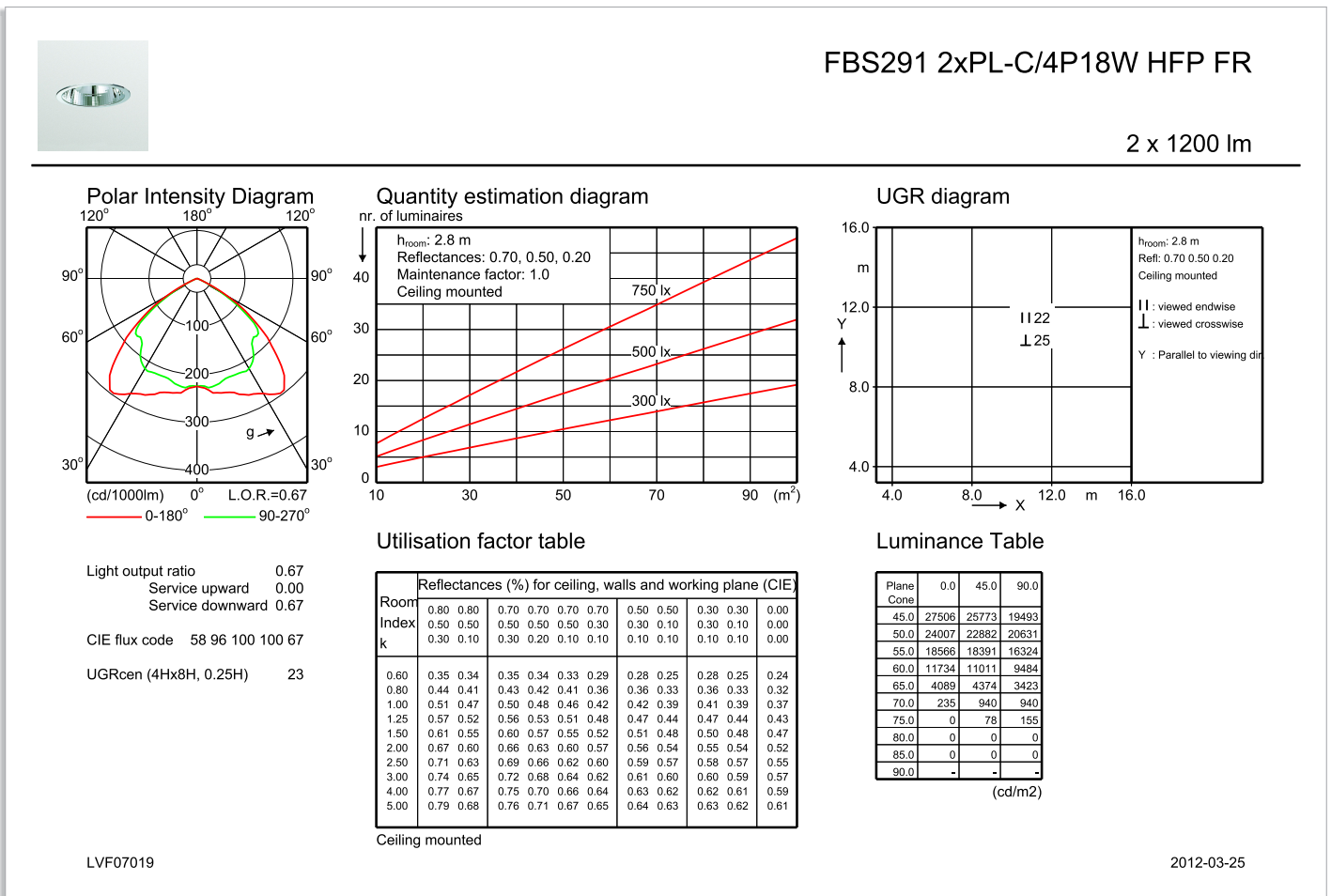
FBS291 2xPL-C/4P18W HFP FR
