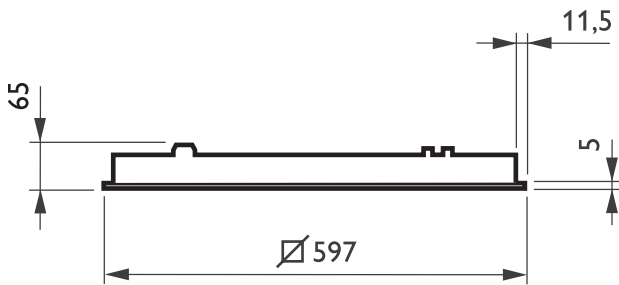
TBS464 3x14W/830 HFP SQR D8-C W IPD-BL
