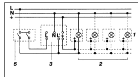
3. Anslutning via strömställare för manuell och automatisk drift
