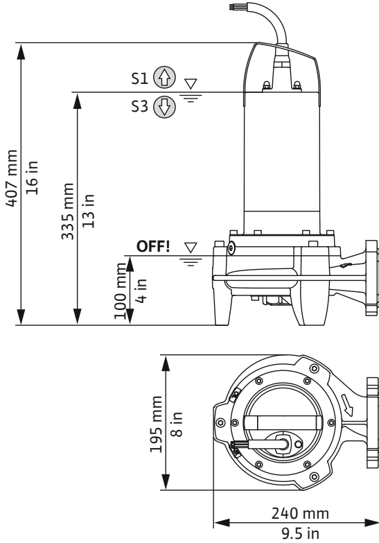
Fig. 3: Asennusmitat
