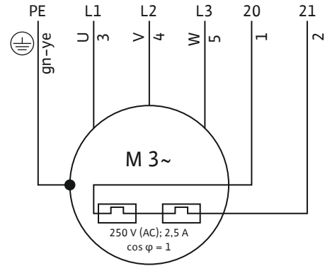
Fig. 5: Liitântäkaavio 3~moottori
