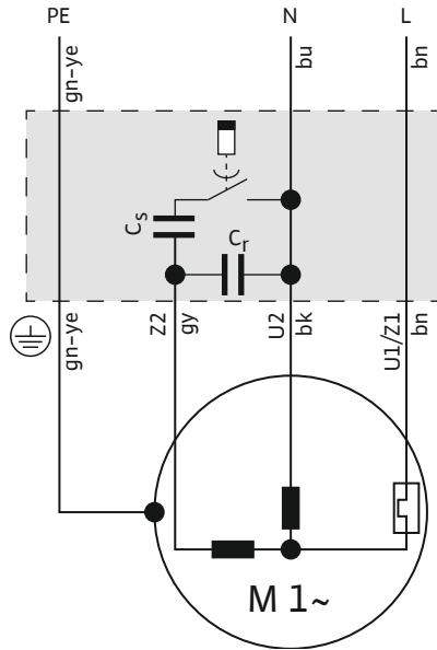
Fig. 4: Liitântäkaavio 1~moottori
