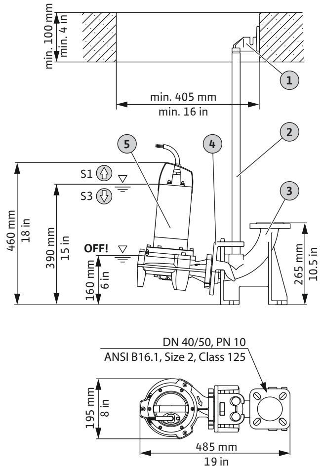
Fig. 2: Osien ja asennusmittojen yleiskatsaus
