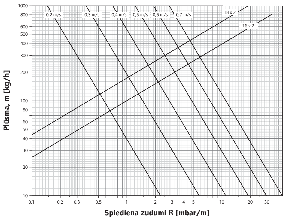
Spiediena zudumu diagramma Uponor daudzslāņu caurulei
