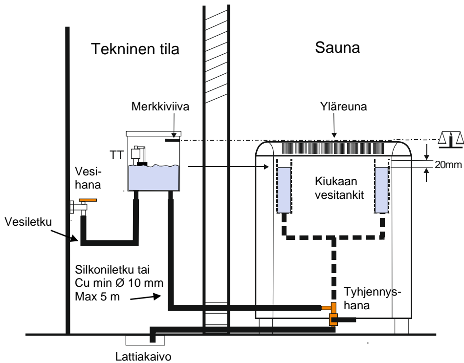
Tasaustankki asennettu tekniseen tilaan.
