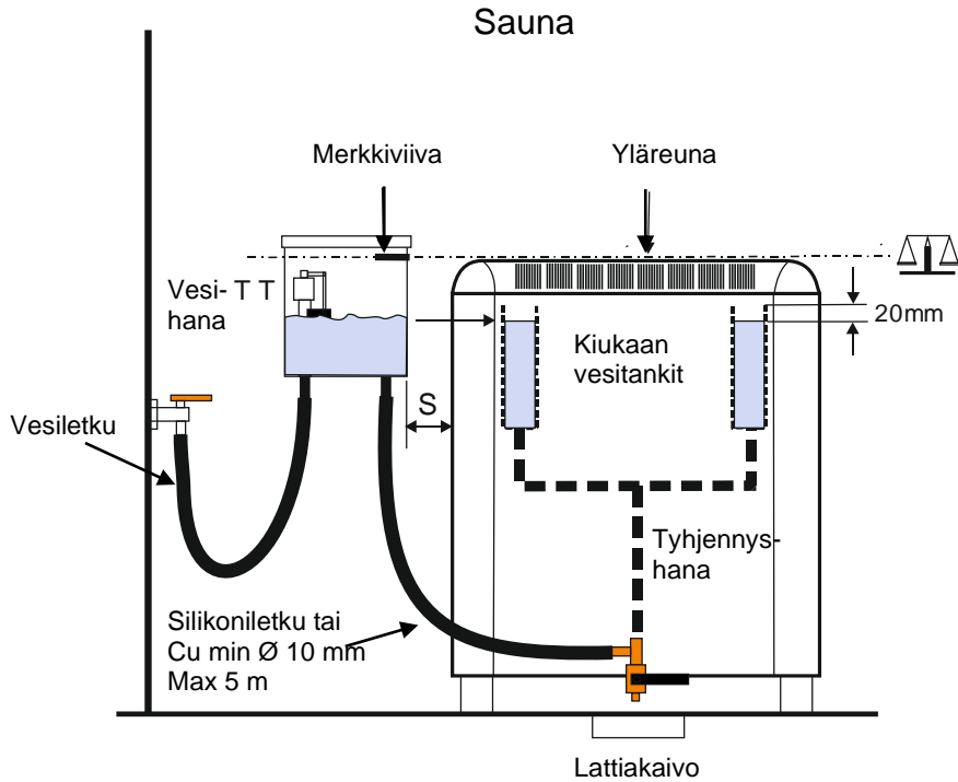
Tasaustankki asennettu saunatilaan
