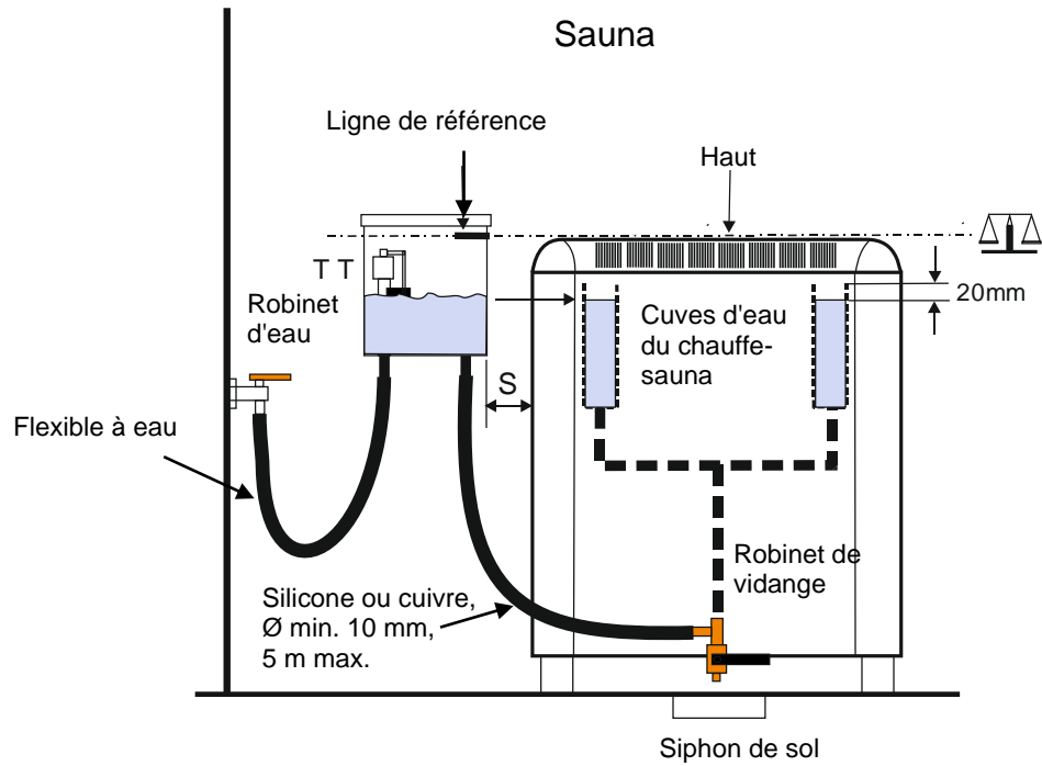
Installation de la cuve de régulation dans la cabine de sauna
