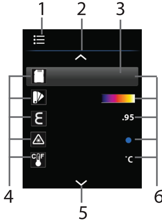
Kuva 9-2 Päävalikossa navigointi
