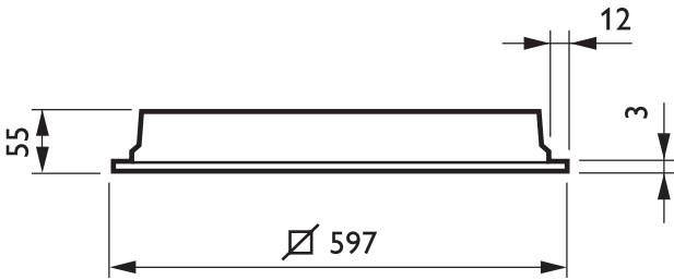
TBS260 3xTL5-14W/830 HFS D6 PI
