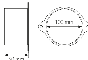
Vastakappale VKP-100
