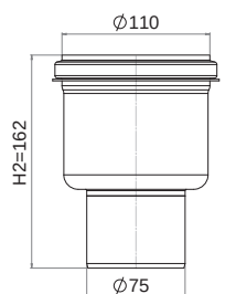
Brunnsdel Bottenutlopp Ø75
