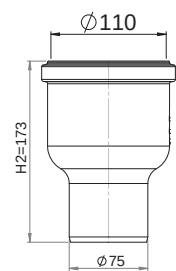
Brunnsdel Bottenutlopp Ø75
