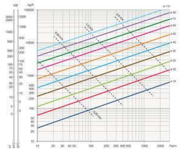
Painehäviötaulukko - Lämpöjohdot PN6
