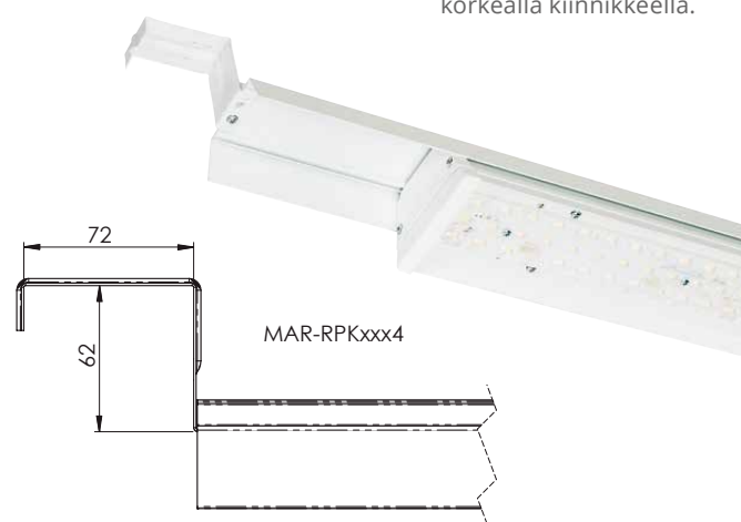
Päätykannake + stoppari 4
