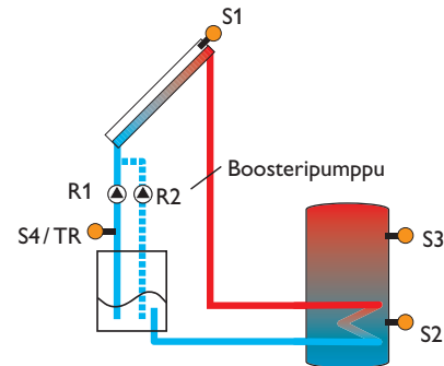
Esimerkkiaavio drainback-järjestelmälle (R2 = boosteripumppu)
