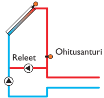
Vaihtoehto pumppu:
