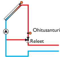
Vaihtoehto venttiili:
