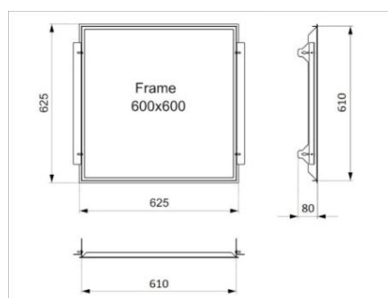
Asennuskehys kipsilevykattoon 600x600
