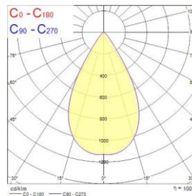
229W 4000K 60°
