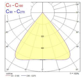
229W 4000K 80°
