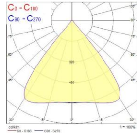
195W 6500K 80°
