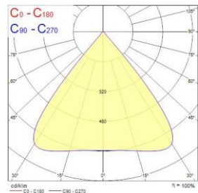
229W 6500K 80°
