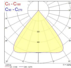
195W 4000K 80°
